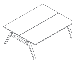
V220 2000 / 1610 / 740 176.2 kg
