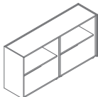
V27 1628 / 424 / 807 79 kg
